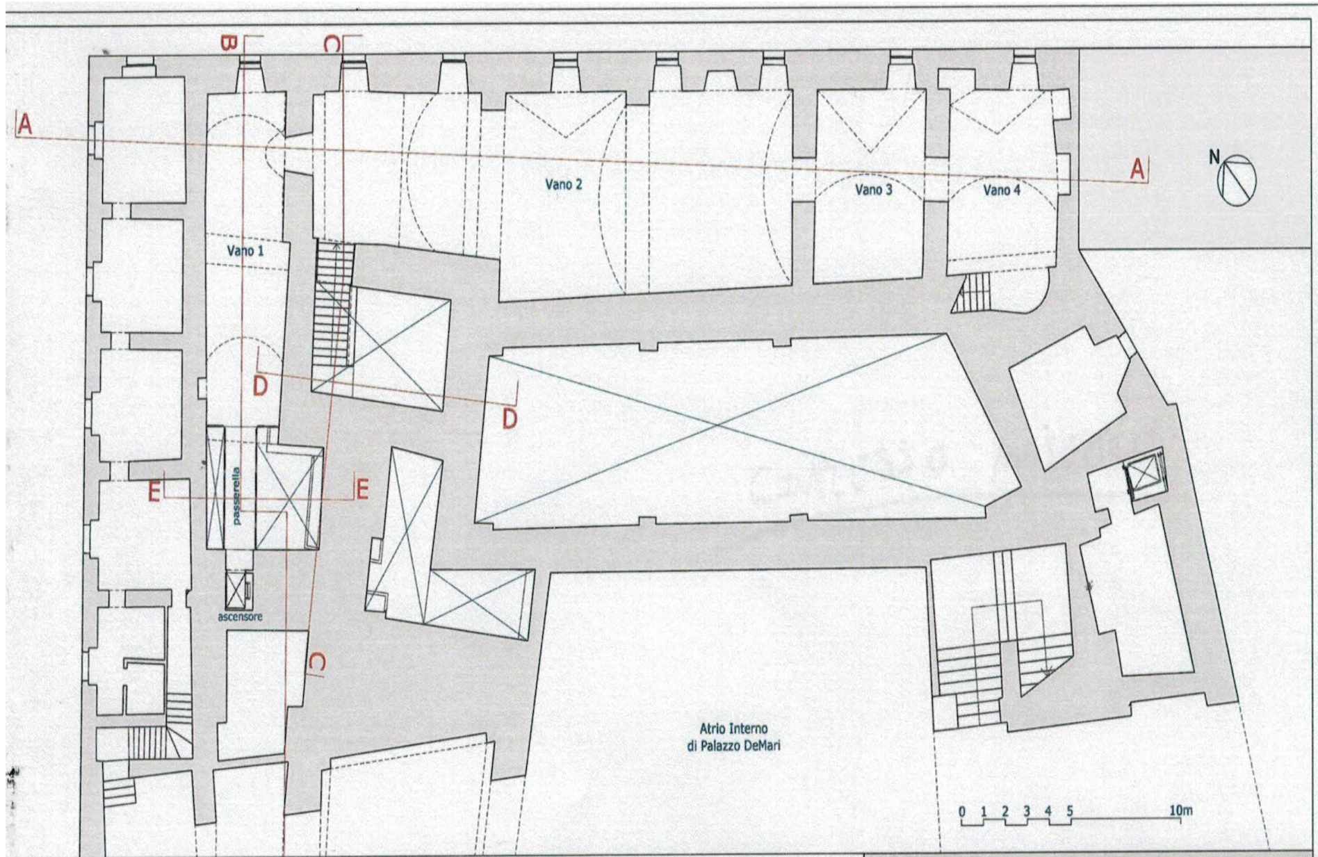
RILIEVO DELLO STATO DEI LUOGHI. Pianta del Piano Ammezzato (scala 1:100)
